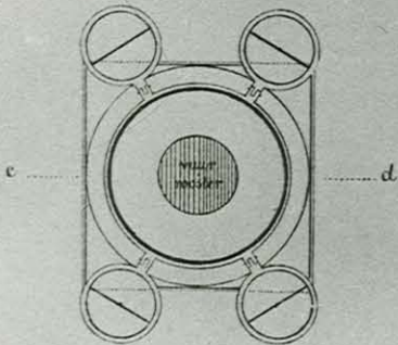
Doorsnede over A. B. fig 1
